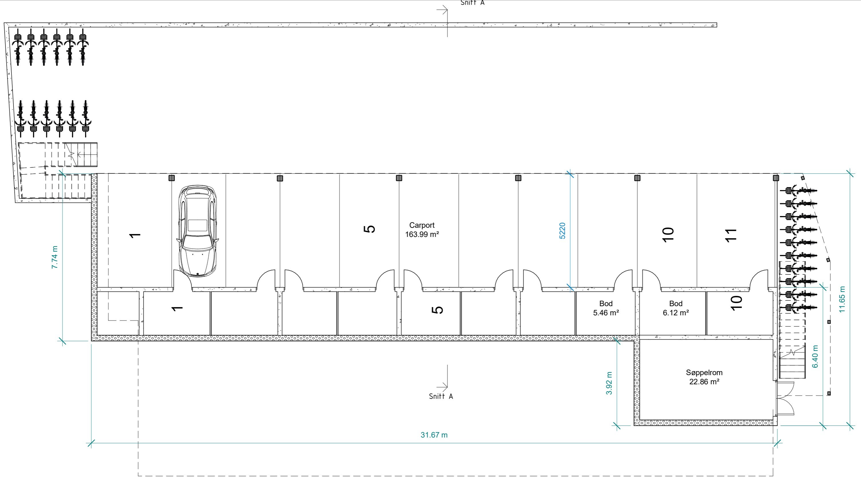
Plan 01 1 : 100
