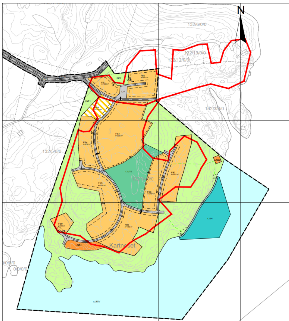
Figur 14 - Utsnitt av reguleringsplan. Rød linje illustrerer formålet for fritidsbebyggelse i dagens KPA. Kilde: Norconsult AS.
