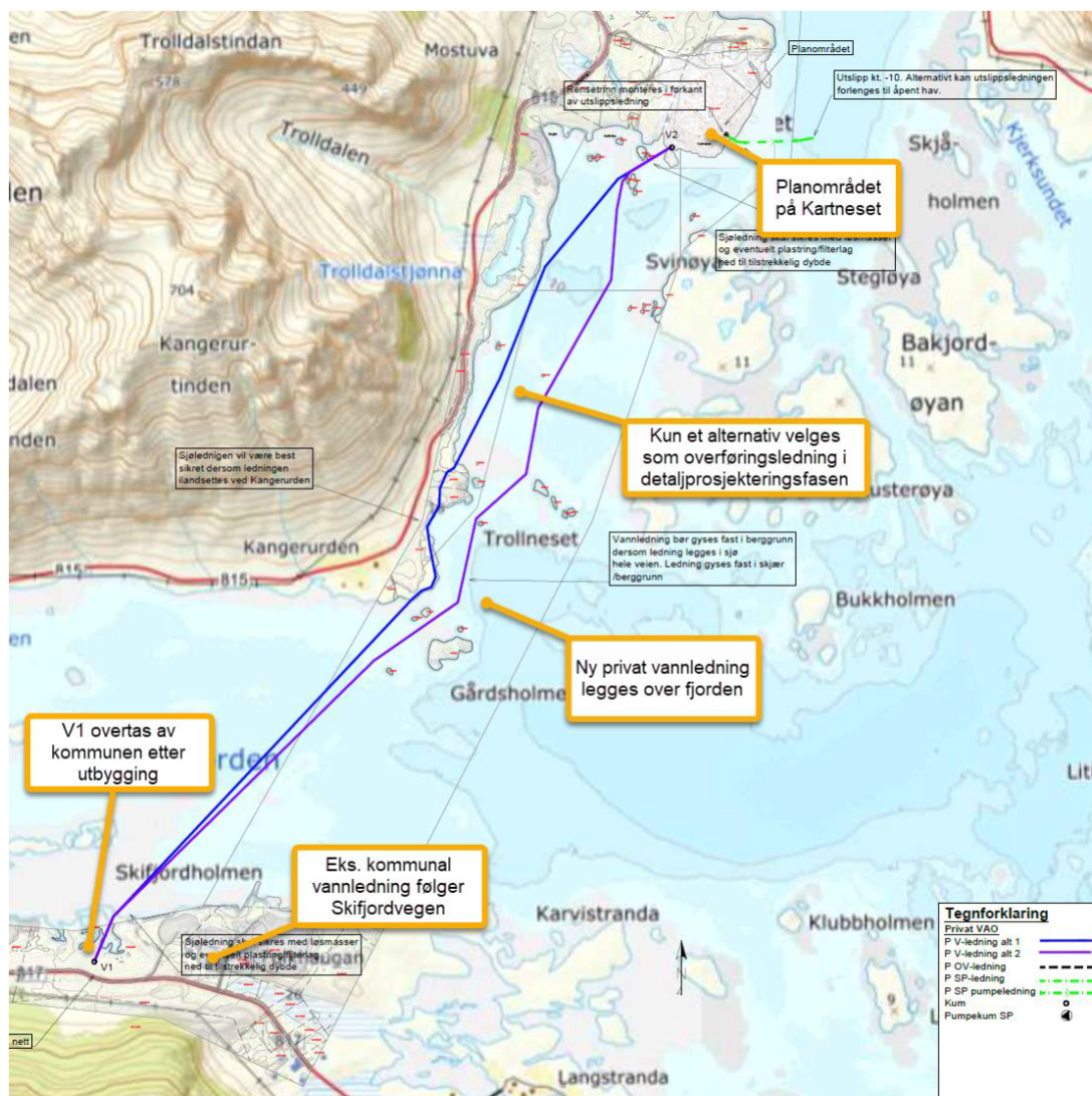
Figur 16 - Privat og kommunalt grensesnitt. Blå linje - alt. 1, lilla linje - alt. 2. Kilde: Norconsult AS.
