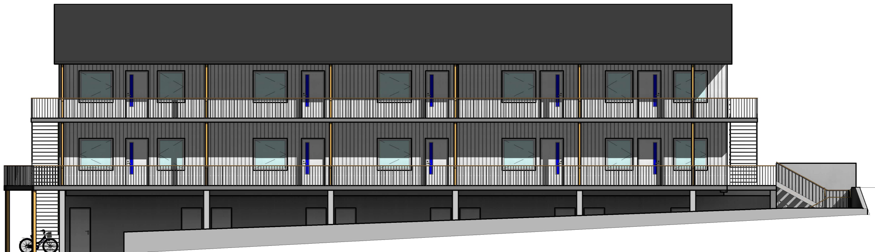
Fasade Øst 1 : 100
