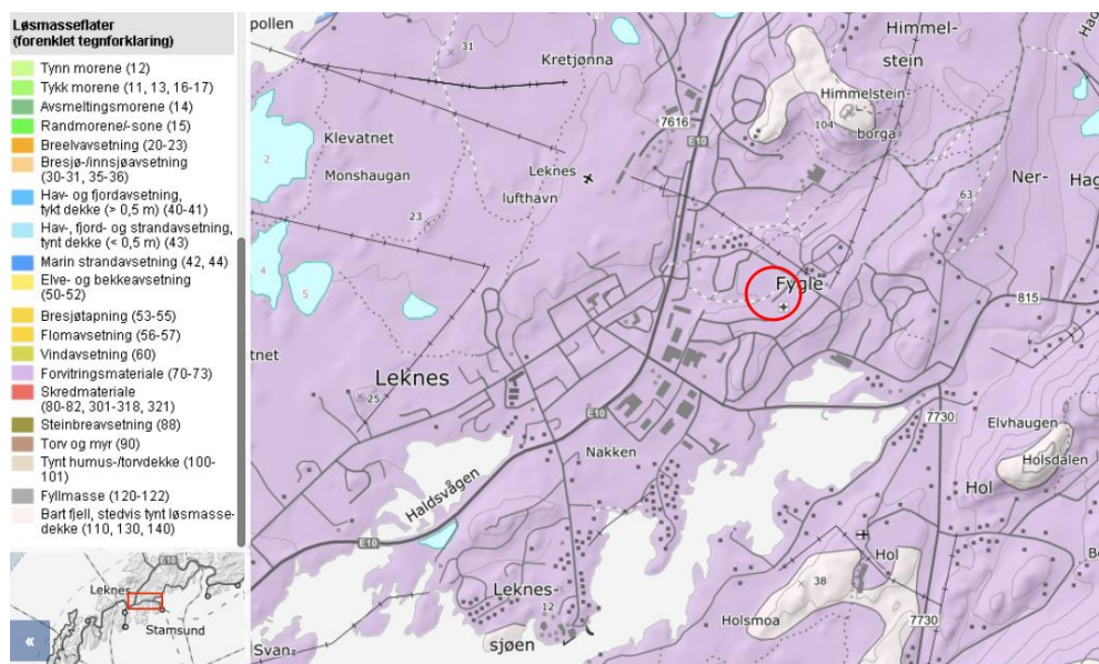
Fig 3: kvartærgeologisk kart. [ngu.no]
