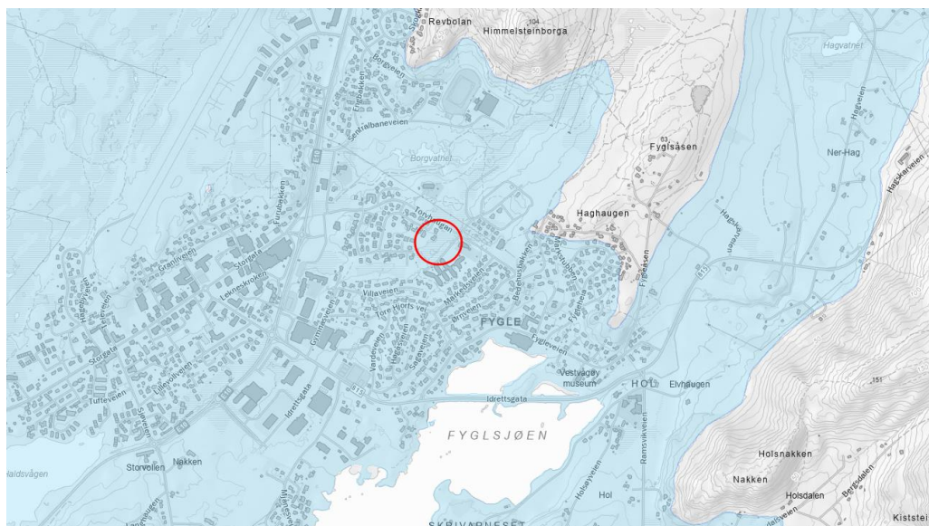
Fig 4: Aktsomhetsområde for marin leire [atlas.nve.no]
