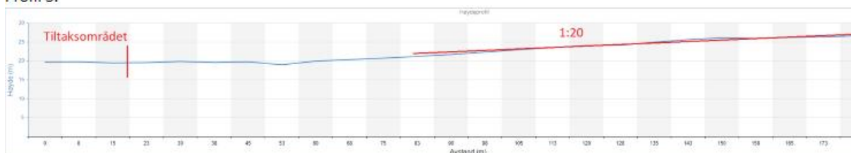
Fig 5: Plan og profil over aktsomhetsområde [atlas.nve.no]
